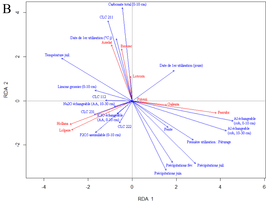
Figure 18 Projections des présences (A) et des abondances (B) des espèces les mieux prédites et des critères sélectionnés. Le détail des corrélations entre axes et critères, et entre axes et espèces est présenté en (Annexe 7)
